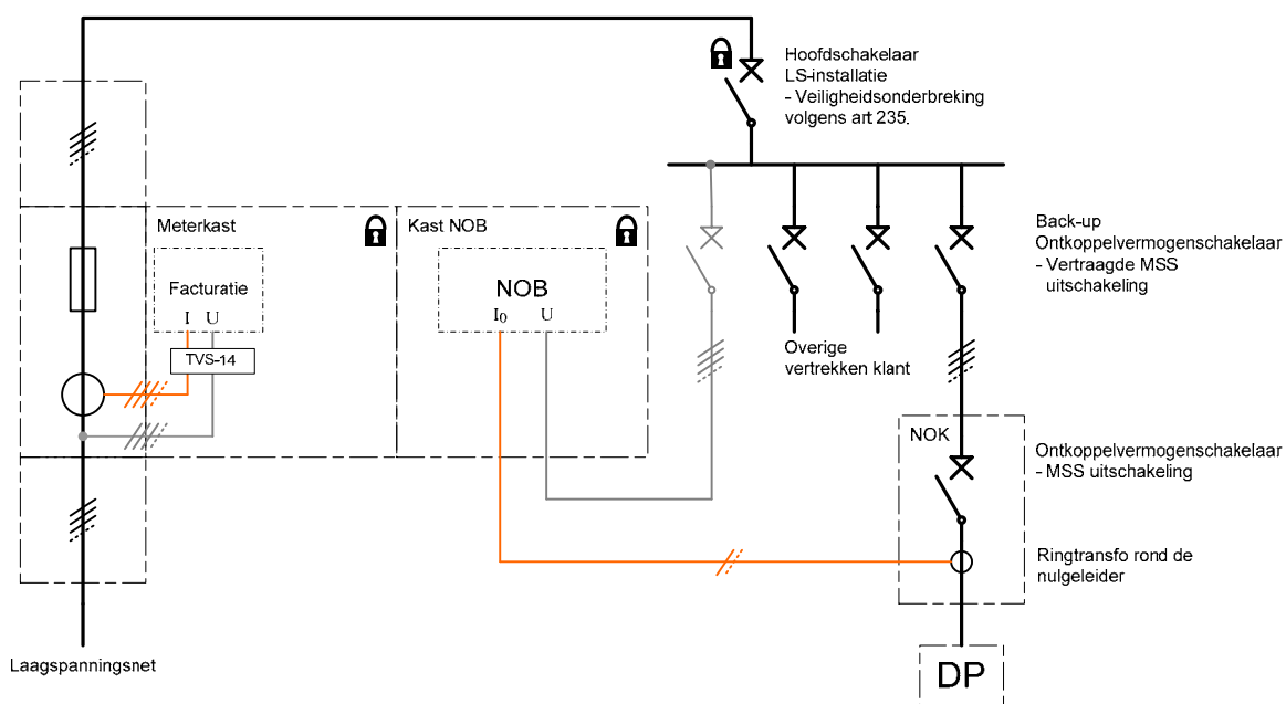
Figuur 1: Krachtinstallatie netontkoppelbeveiliging van een installatie voor decentrale productie van klantinstallaties op het LS distributienet
